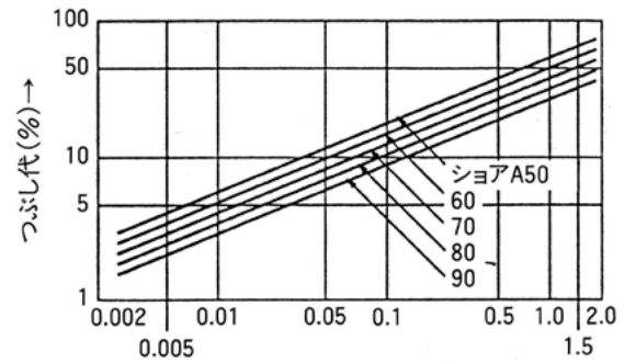
図7 Oリングのつぶし代とつぶし力
