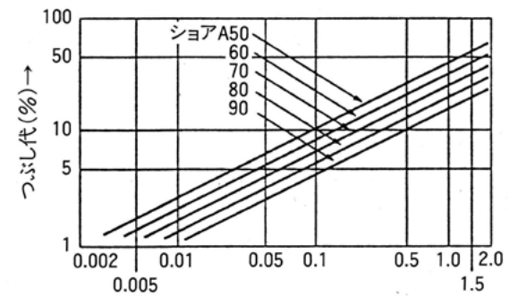
図9 Oリングのつぶし代とつぶし力
