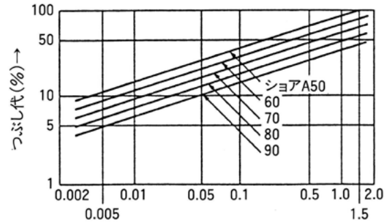
図5 Oリングのつぶし代とつぶし力
