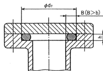
図12 内圧用 (Oリングが内側に引込まれない場合)
