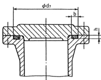
図11 内圧用
