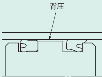
図10 背圧発生によりピストンパッキンがかみ込んだところ
