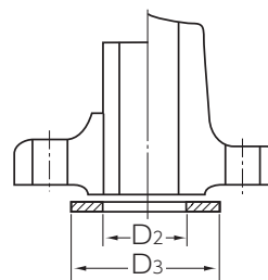
小平面座フランジ用
