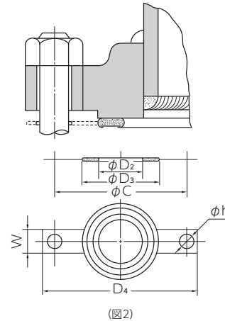
取手付メタルジャケットガasket
