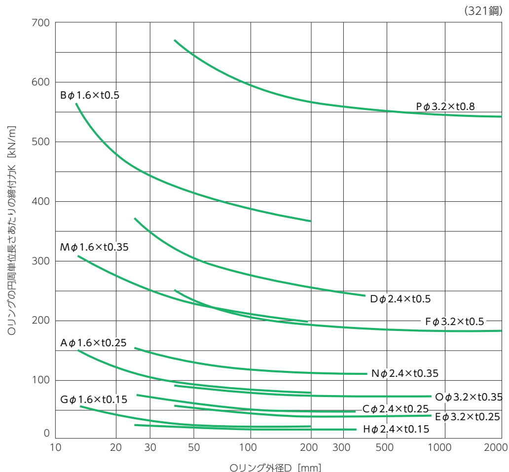
メタル中空リングの円周単位長さあたりの締付力
