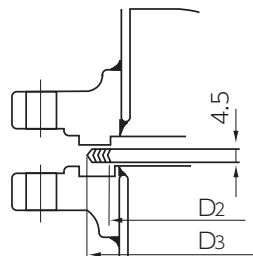
溝形(タング・グループ)フランジ用
